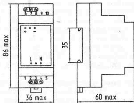
Рис 1. Габаритный чертеж
