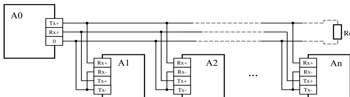
A0 – ведущий абонент; A1...An – ведомые абоненты; Rc – согласующий резистор 470 Ом±10%
