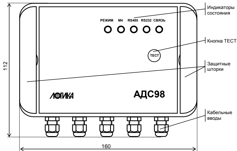
Рисунок 3.1 – Вид спереди
